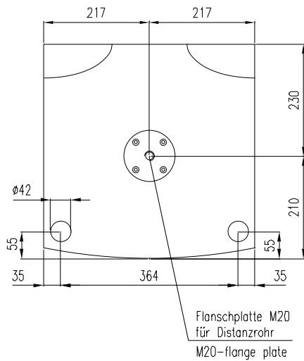
Draufsicht / Top view
