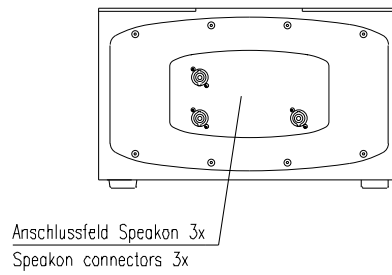
Rückansicht / Rear view
