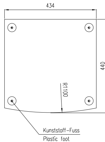
Bodensicht / Bottom view
