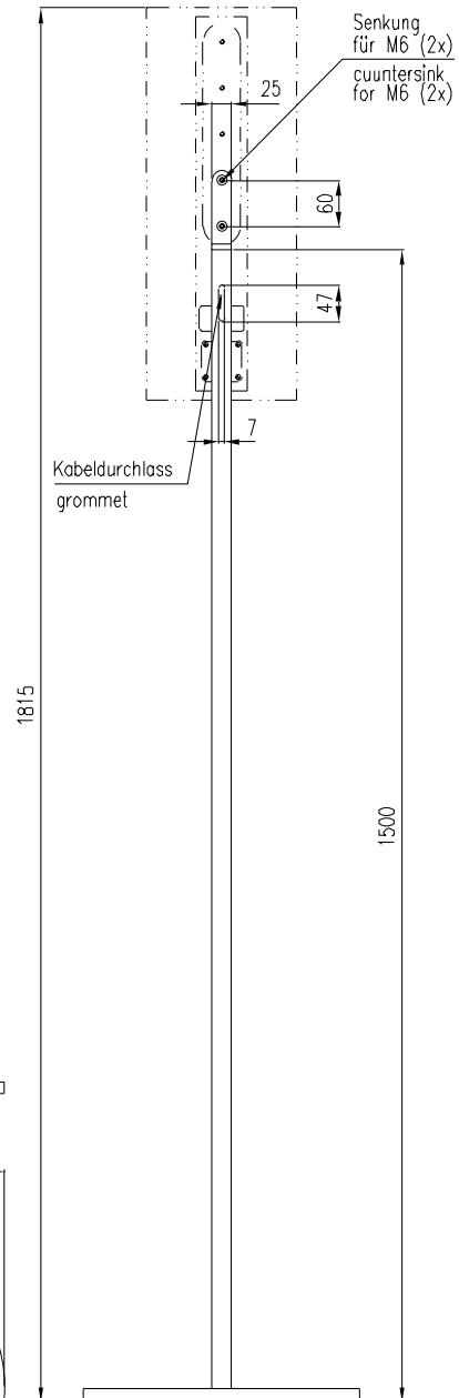
Rückansicht / Rear view
