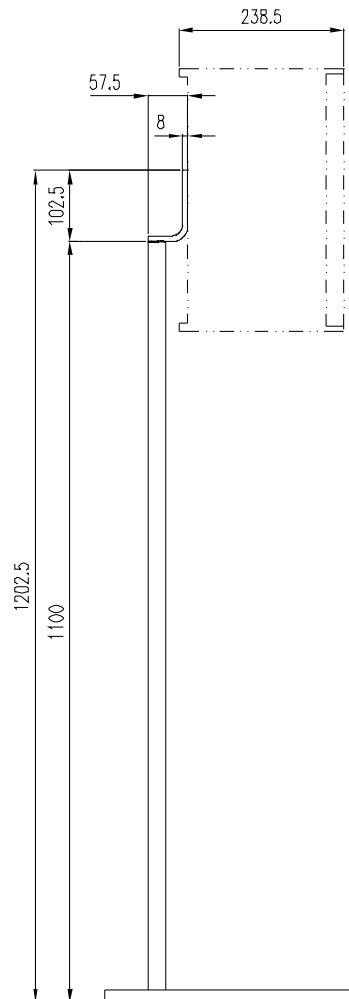
Seitenansicht / Side view
