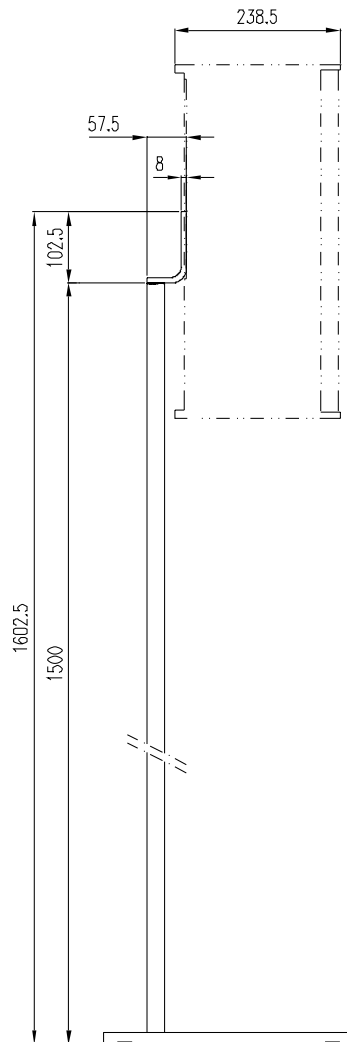
Seitenansicht / Side view
