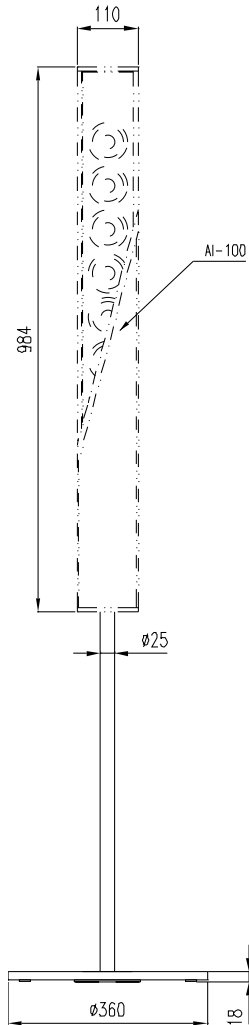
Vorderansicht / Front view
