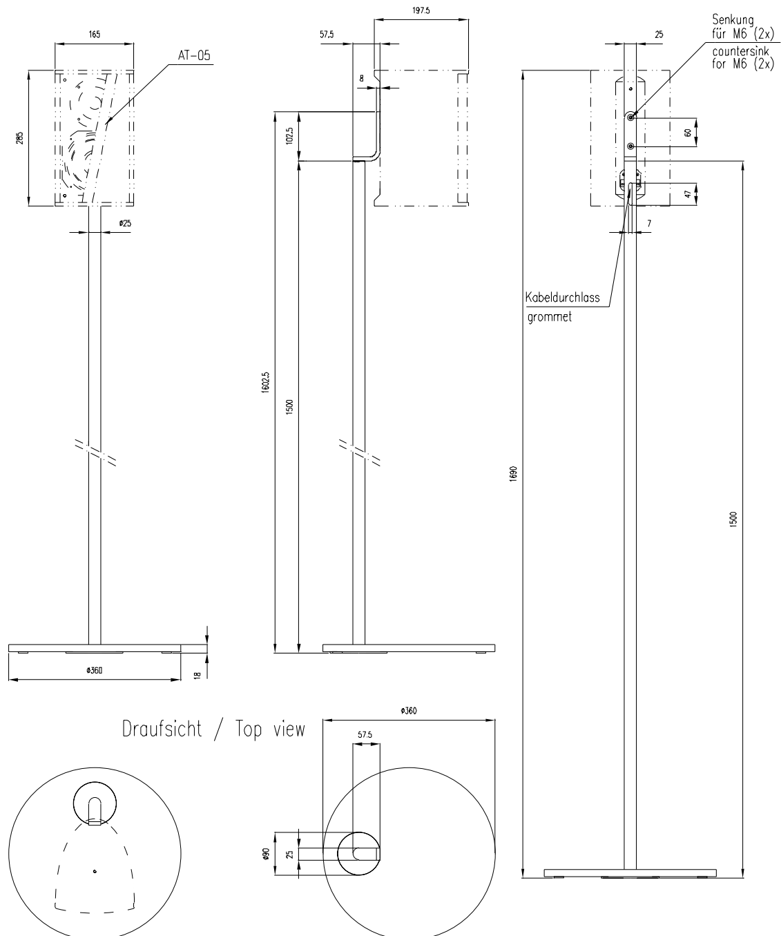
vorderansicht / Front view
