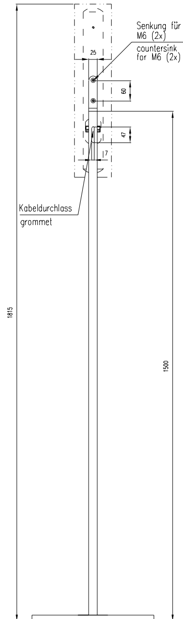
Rückansicht / Rear view
