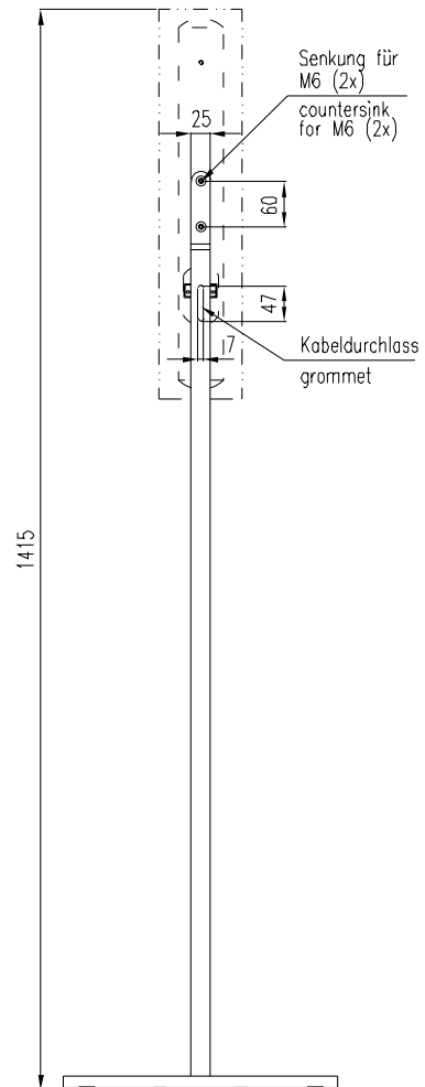
Rückansicht / Rear view
