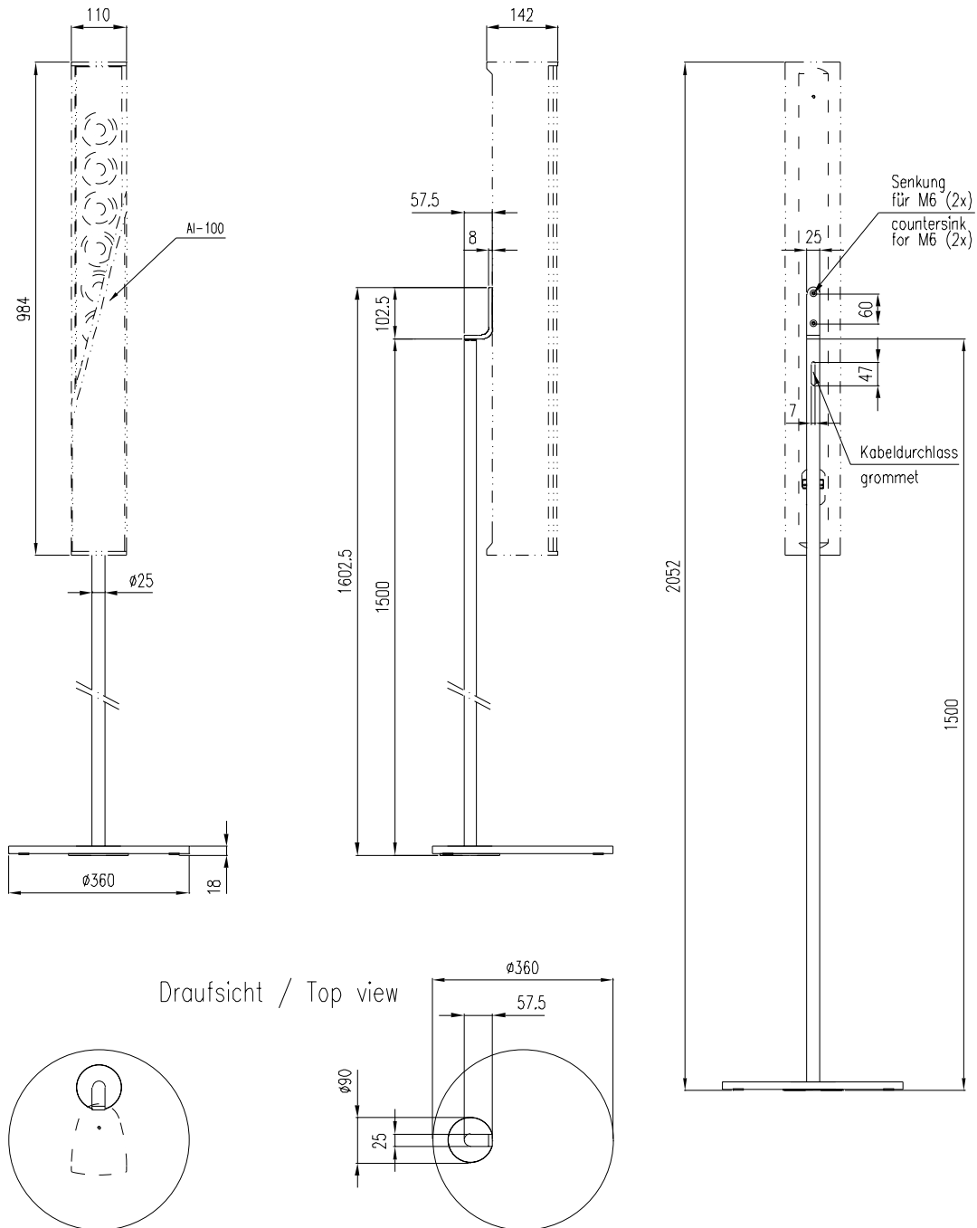
Vorderansicht / Front view
