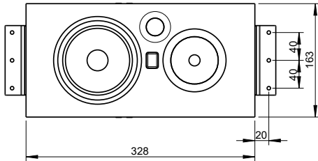
VORDERANSICHT
