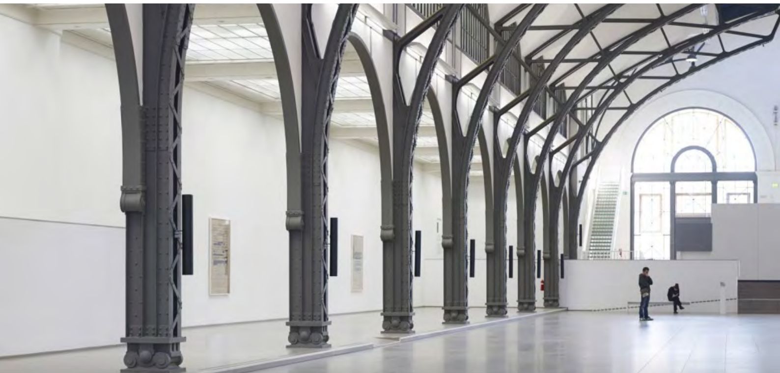
MUSEUM FÜR GEGENWART, BERLIN: Bei einer 24-Kanal-Klanginstallation der Künstlerin Susan Philipsz ließen 24 LINEA LX-100 Linienstrahler (montiert an zwei Säulenreihen) Musikstücke des Komponisten Hanns Eisler regelrecht durch die Halle wandern. Foto: ©Isabella Bortollozi Galerie
