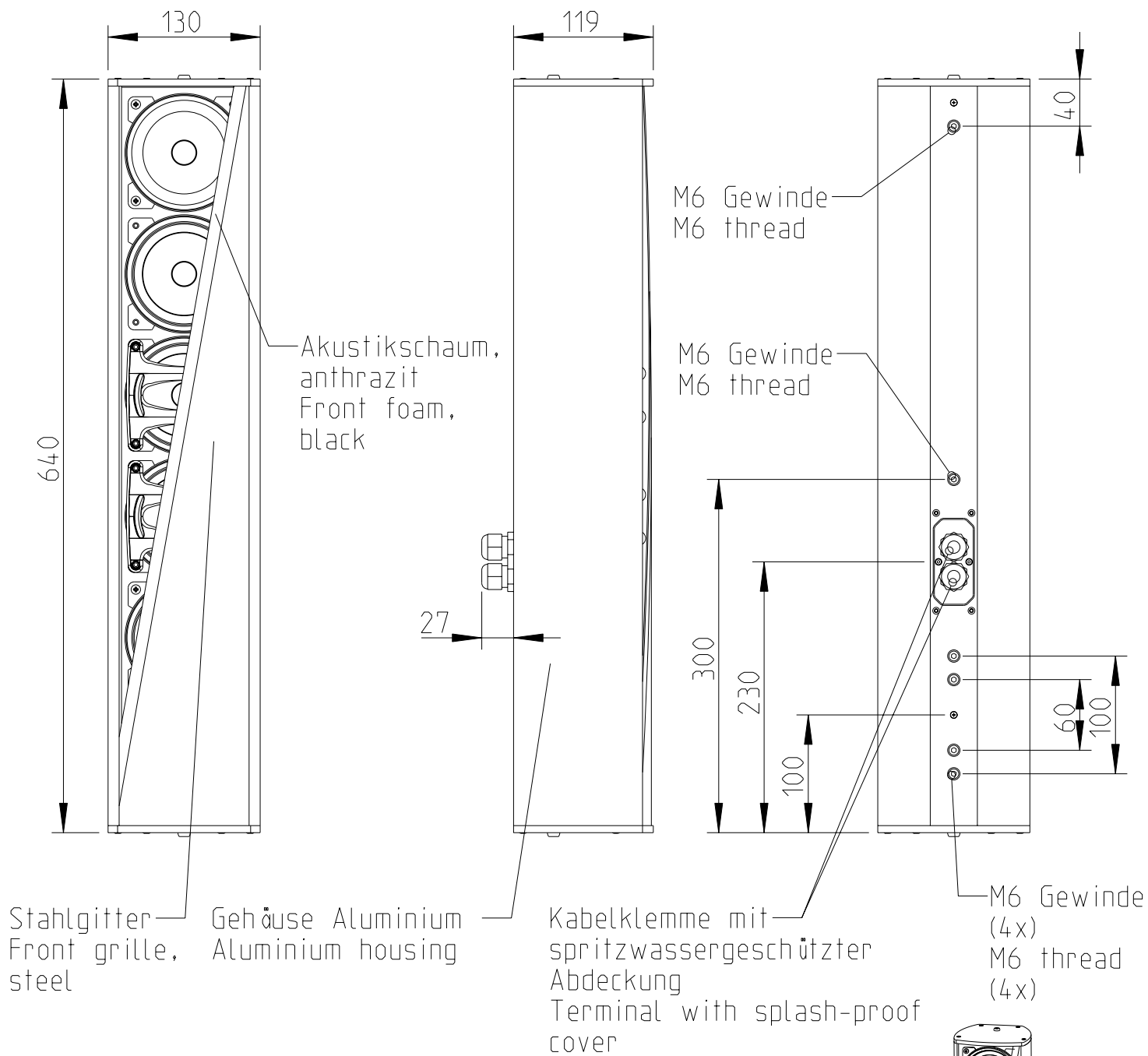
Vorderansicht/ Front view
