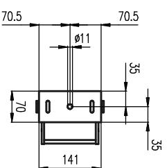
Ansicht X / View X
