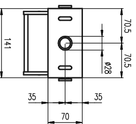
Draufsicht ohne Clamp / Top view without Clamp
