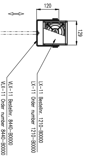
Vorderansicht / Front view
