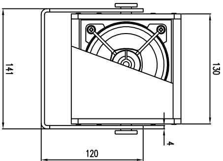
Vorderansicht / Front view
