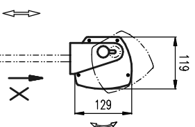
Seitenansicht / Side view
