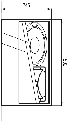
Vorderansicht 35° / Front view 35°
