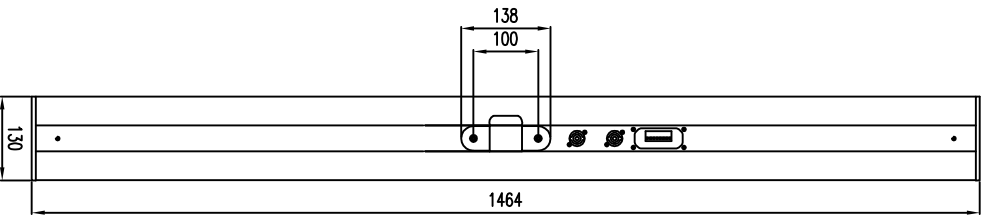
Rückansicht / Rear view
