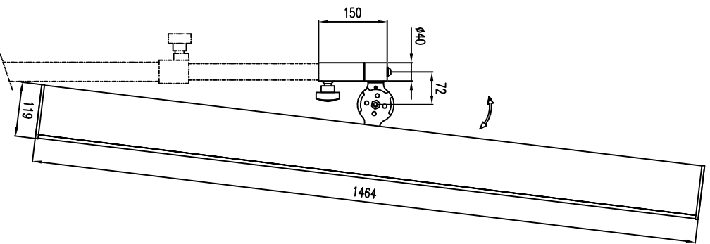
Seitenansicht / Side view
