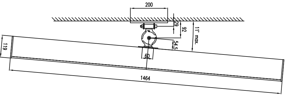
Seitenansicht / Side view
