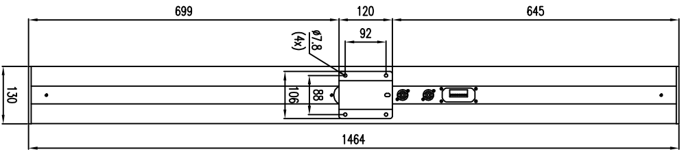
Draufsicht / Top view
