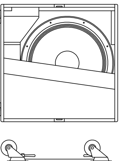
Vorderansicht / Front view
