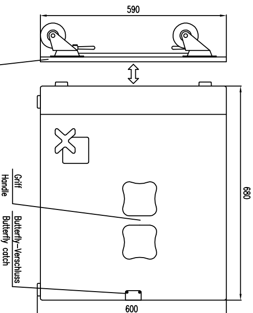
Seitenansicht / Side view
