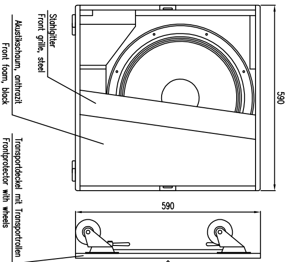
Vorderansicht / Front view
