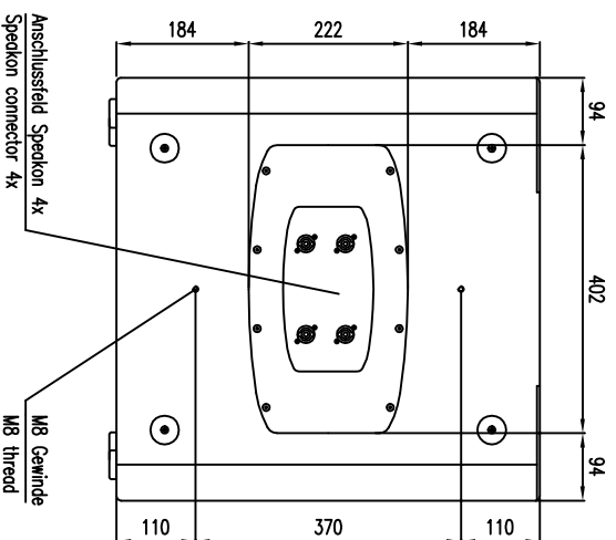
Rückansicht / Rear view
