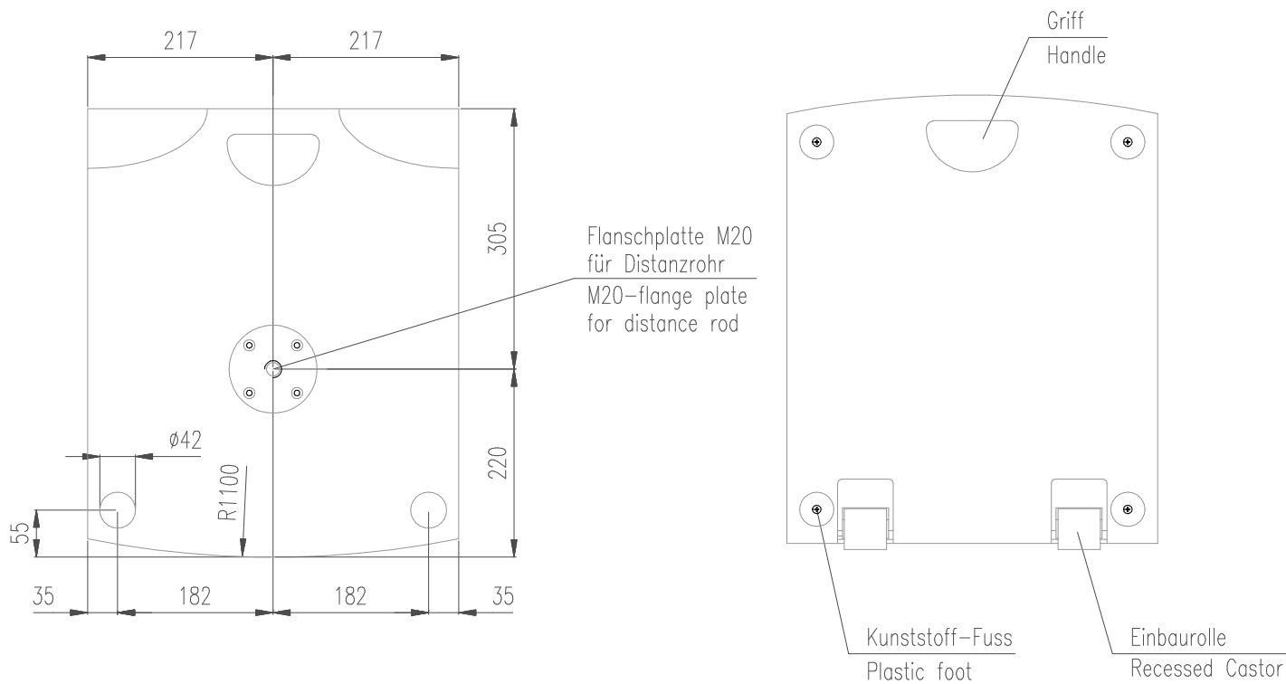
Bodensicht / Bottom view
