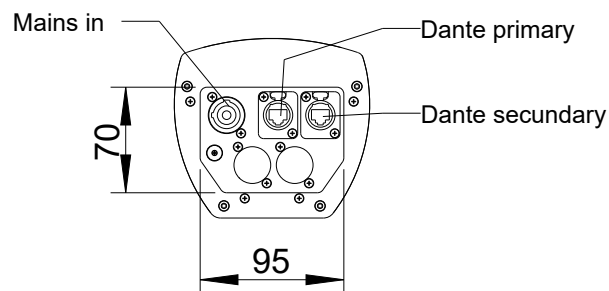
Ansicht von unten/ Bottom view 1:5
