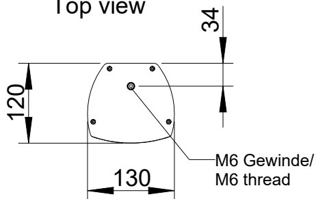
Draufsicht / Top view
