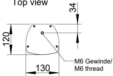
Draufsicht / Top view
