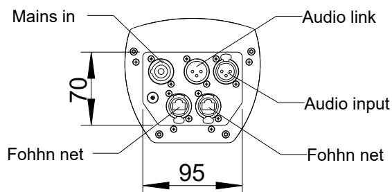
Ansicht von unten/ Bottom view
