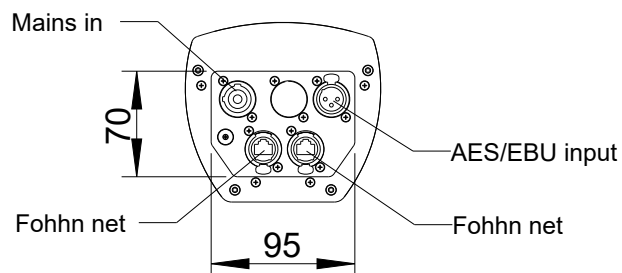
Ansicht von unten / Bottom view 1:5
