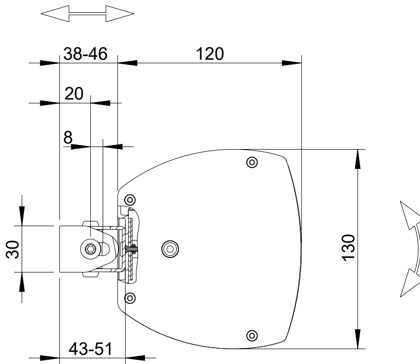
Draufsicht / Top view
