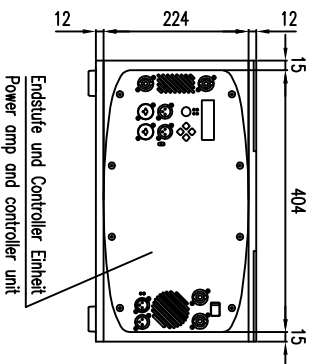
Rückansicht / Rear view
