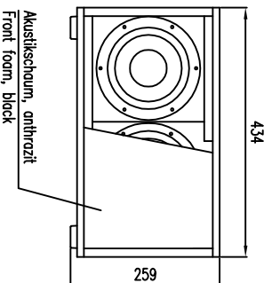
Vorderansicht / Front view
