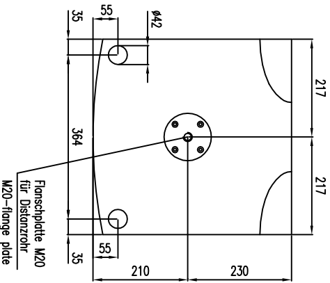
Draufsicht / Top view
