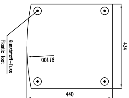
Bodensicht / Bottom view
