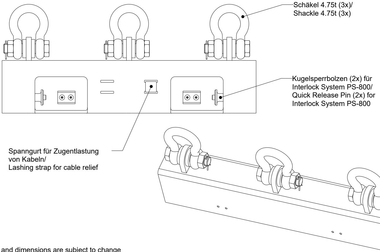
Rückansicht / Rear view
