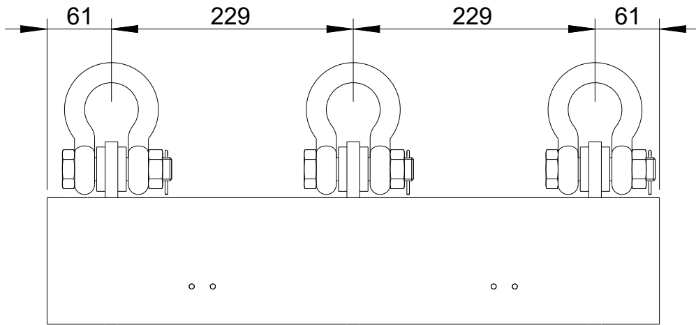
Draufsicht / Top view
