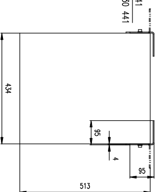
Draufsicht V. 3 u. 4 / Top view V. 3 u. 4
