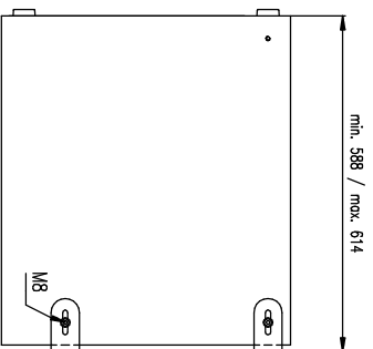
Draufsicht / Top view Variante 1 / Variation 1
