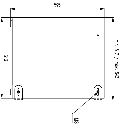
Rückansicht / Rear view Variante 3 / Variation 3
