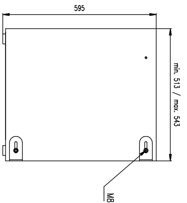
Rückansicht / Rear view Variante 4 / Variation 4
