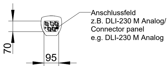
Ansicht von unten/ Bottom view
