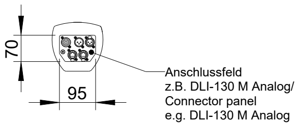
Ansicht von unten/ Bottom view
