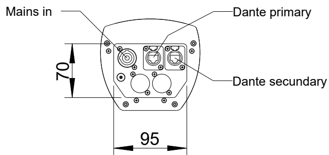
Ansicht von unten/ Bottom view 1:5
