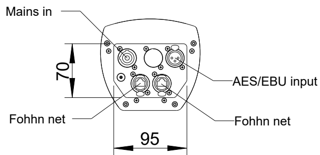
Ansicht von unten/ Bottom view 1:5
