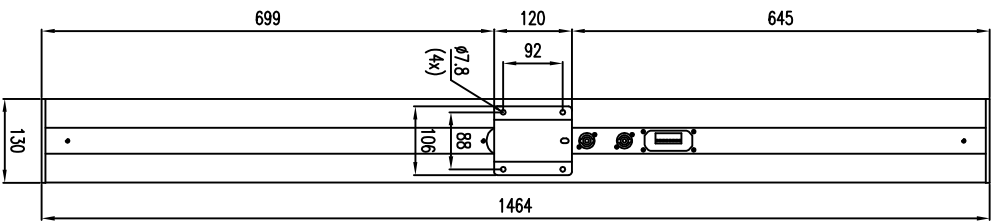
Draufsicht / Top view
