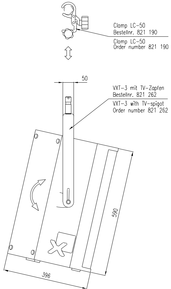
Seitenansicht / Side view
