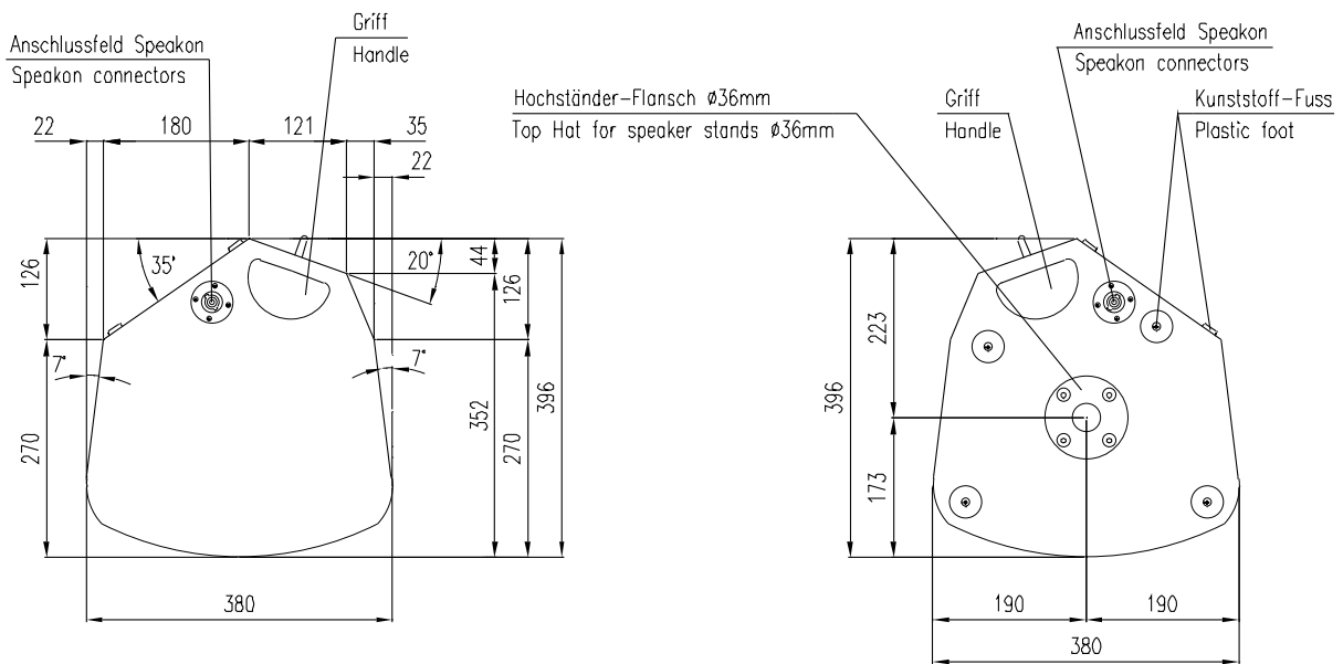
Draufsicht / Top view
