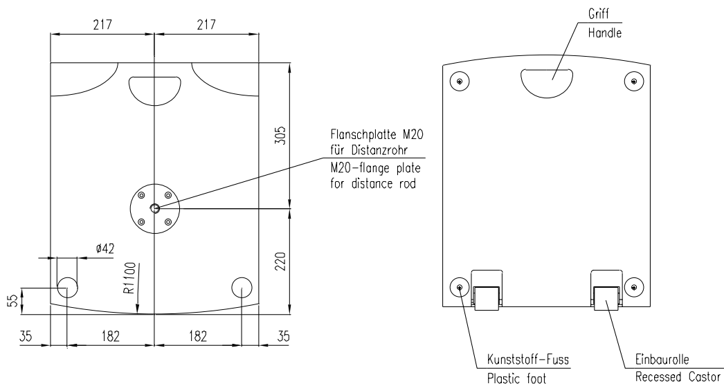
Draufsicht / Top view
