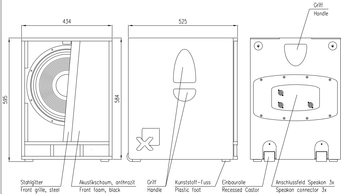
Vorderansicht / Front view
