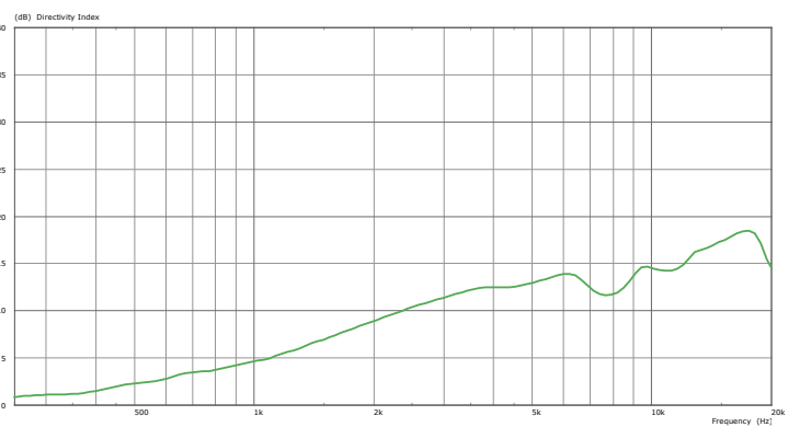
Bild 5: Bündelungsmaß
