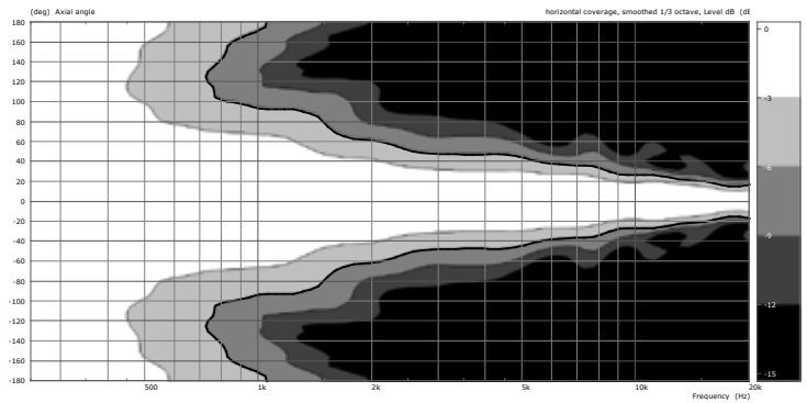
Bild 2: Isobaren horizontal
