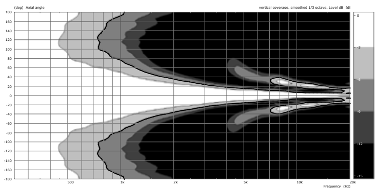
Bild 4: Isobaren vertikal
